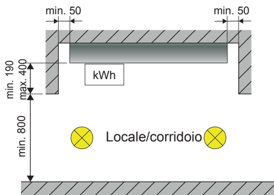
Montaggio in nicchia
