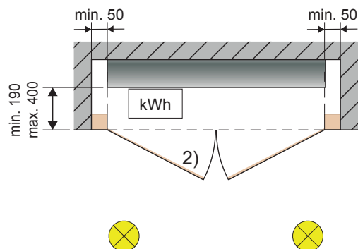
Montaggio in armadio
